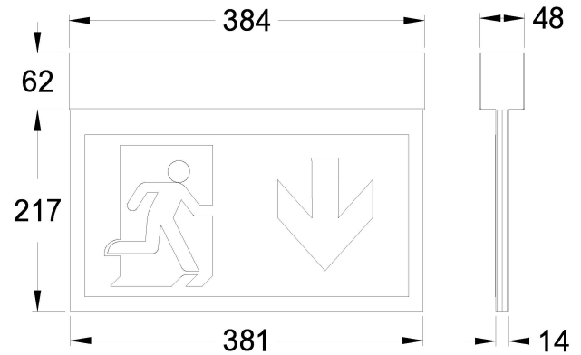
Maßzeichnung (Angaben in mm)
