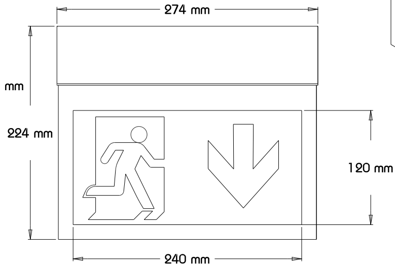
Ansicht Hinten
