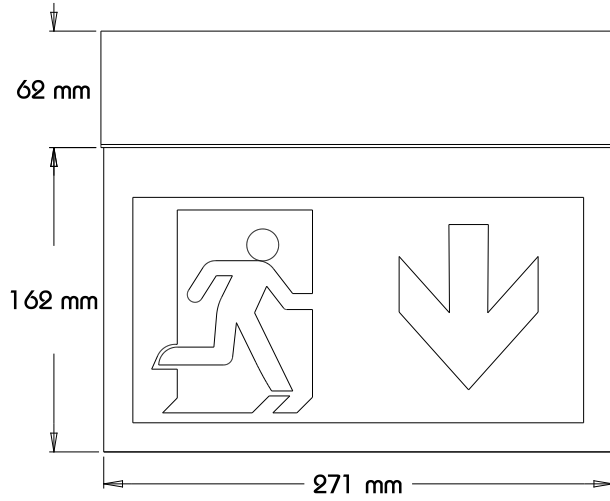
Ansicht Vorne
