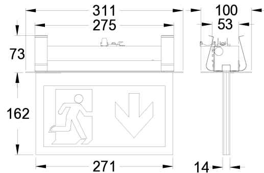
Maßzeichnung (Angaben in mm)
