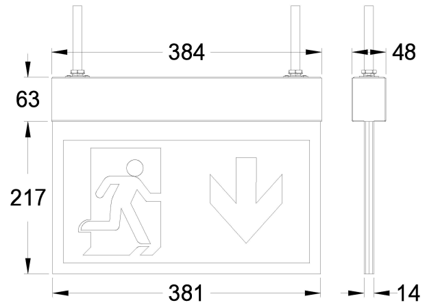
Maßzeichnung (Angaben in mm)
