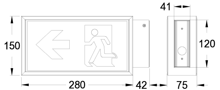
Maßzeichnung (Angaben in mm)
