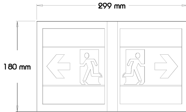
Ansicht Vorne
