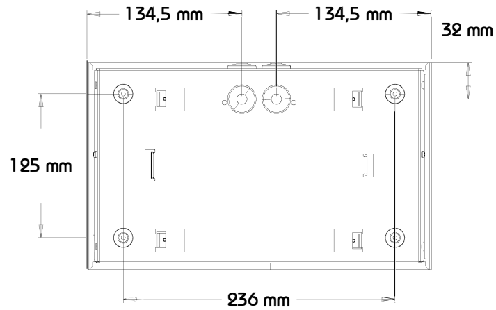
Ansicht Hinten
