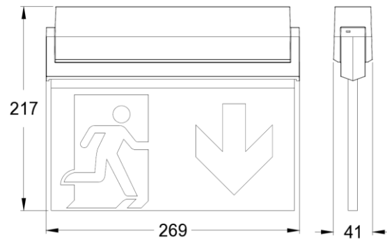
Maßzeichnung (Angaben in mm)
