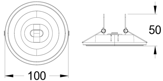
Maßzeichnung (Angaben in mm)
