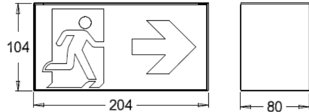
Maßzeichnung (Angaben in mm)
