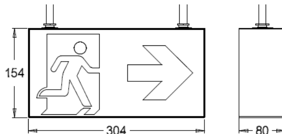
Maßzeichnung (Angaben in mm)
