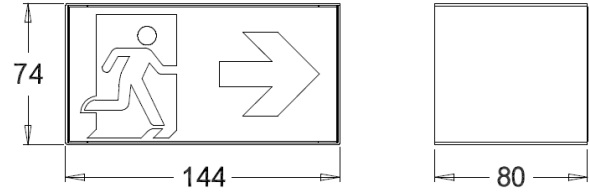
Maßzeichnung (Angaben in mm)
