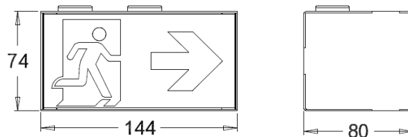
Maßzeichnung (Angaben in mm)
