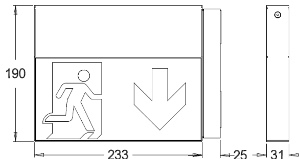
Maßzeichnung (Angaben in mm)
