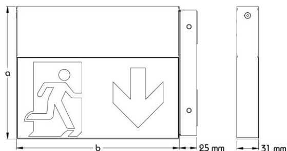
Maßzeichnung
