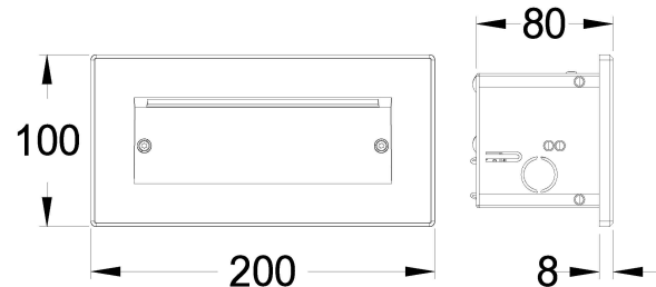
Maßzeichnung
