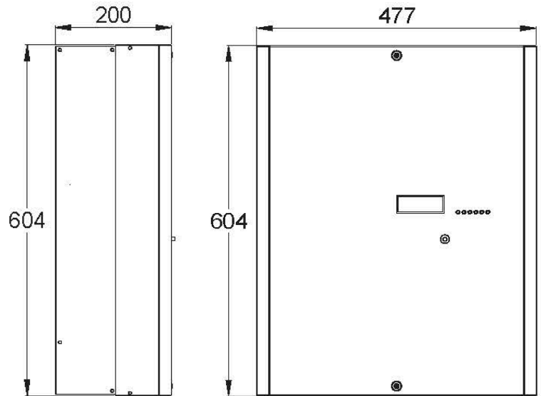
Maßzeichnung (Angaben in mm)
